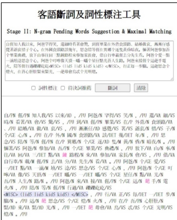
圖 13. 斷詞及詞性標注器 (第二階段)
